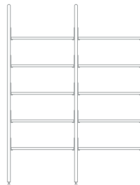
Branch-2 Shelving Unit W64.5 D11.5 H84 (in) W164 D29 H213 (cm)
