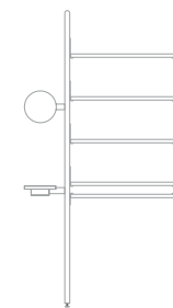
Branch-1 Display Unit W48.5 D11.5 H84 (in) W123 D29 H213 (cm)
