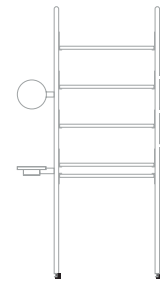
Branch-1 Display Unit W48.5 D11.5 H84 (in) W123 D29 H213 (cm)
